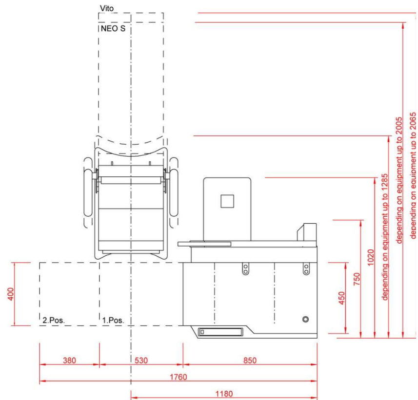
Abbildung 16: Untersuchungseinheit CaraT® rechts Ausführung für zwei Geräte
